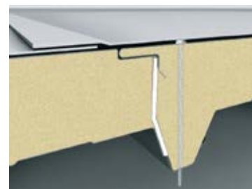
Particolare del giunto Joint detail
